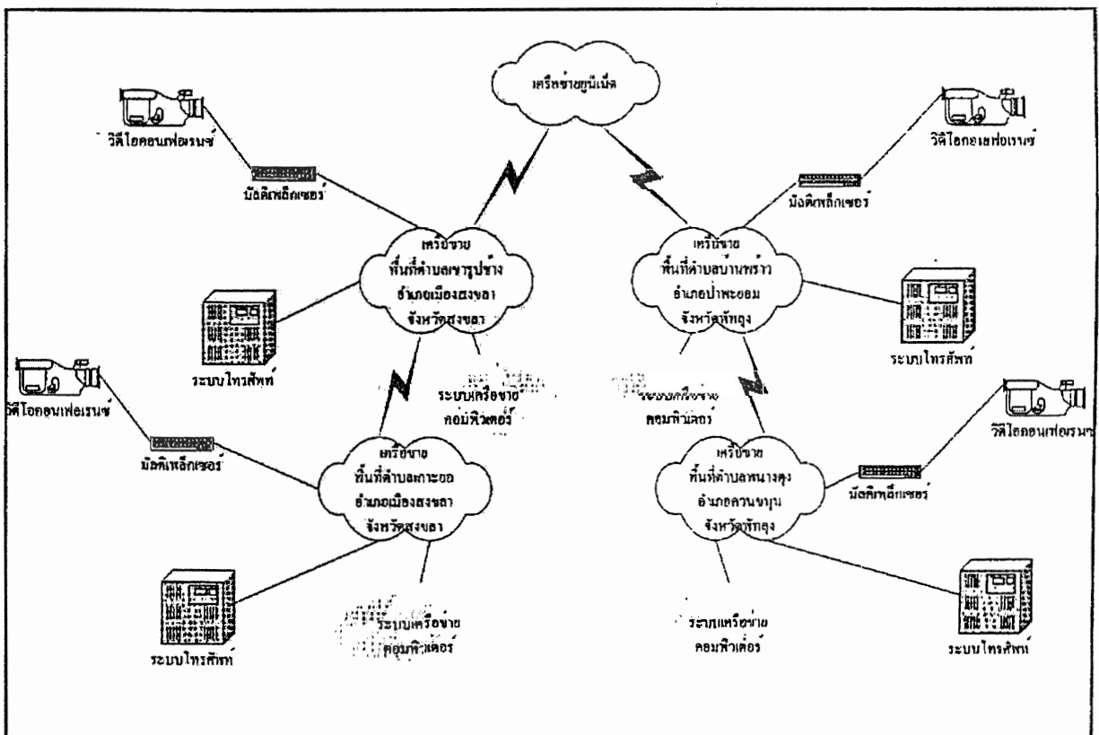
แผนภาพแสดงระบบเครือข่ายมหาวิทยาลัยทักษิณ
