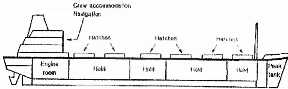
รูปที่ ๔ Single Deck
