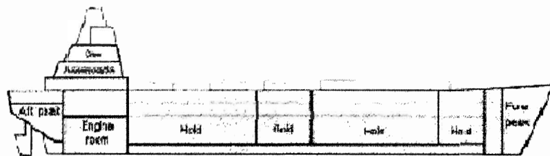
รูปที่ ๒ Gross Tonnage
